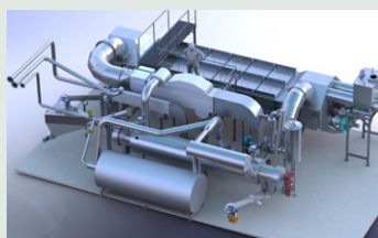
3D tegning af et AquaGreen damp-tørring- og pyrolyseanlæg til behandling af spildevandsslam fra 50.000 personer. Disse anlæg etableres hos Odsherred Forsyning og VandCenter Syd (Nordfyn) i løbet af 2021.
