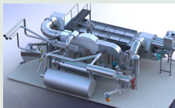
3D tegning af et AquaGreen damp-tørring- og pyrolyseanlæg til behandling af spildevandsslam fra 50.000 personer. Disse anlæg etableres hos Odsherred Forsyning og VandCenter Syd (Nordfyn) i løbet af 2021.
